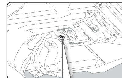
Einstellschraube für Bremsweg
