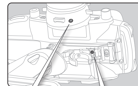
Einstellschraube für Federspannung am Lenkrad
